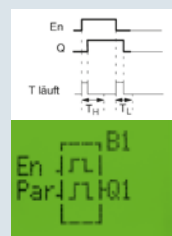
Losowy generator impulsów
