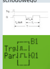
Sterownik oświetlenia schodowego
